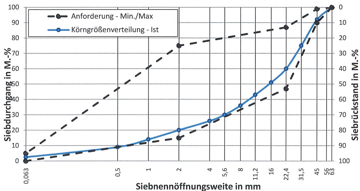
Baustoffgemisch 0/45 für Frostschutzschichten
